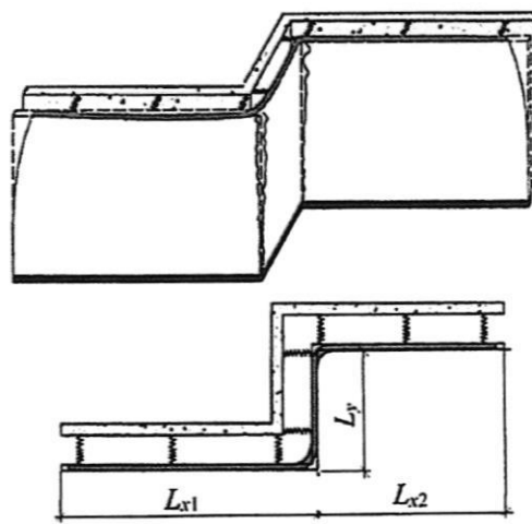
Рисунок В.2 – Схема деформаций лицевого слоя на Z-образном участке в холодное время при его возведении в теплое время
