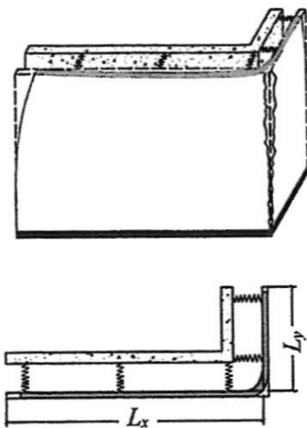
Рисунок В.1 – Схема деформаций лицевого слоя на Г-образном участке с внешним углом в холодное время при его возведении в теплое время
